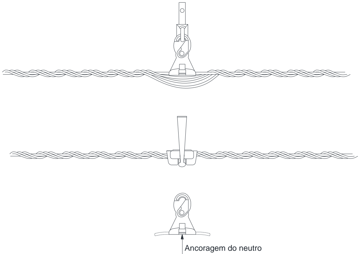
Figura 38 – Amarrações e ligações – Estrutura secundária – Tangente
