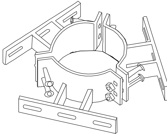
Figura 129 Suporte para equipamento tipo IV
