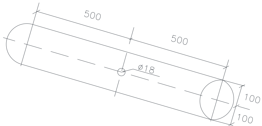
Figura 103 - Morto
