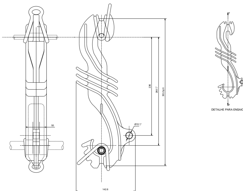
Figura 71 - Espaçador monofásico
