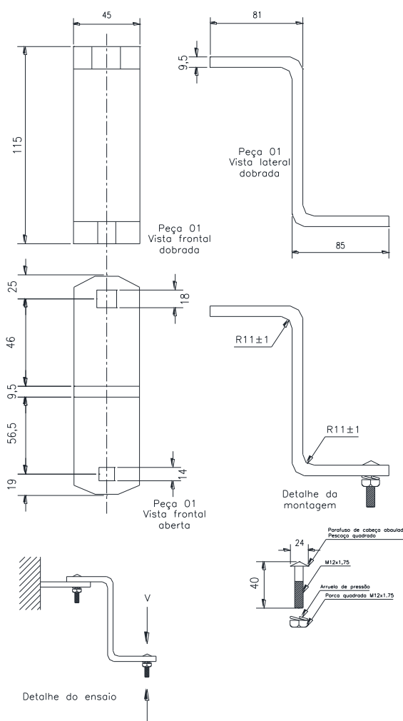
Figura 136 - Suporte Z
