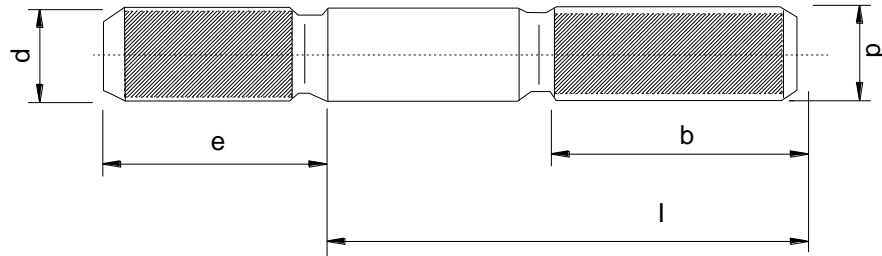
Figura 109 - Parafuso prisioneiro
