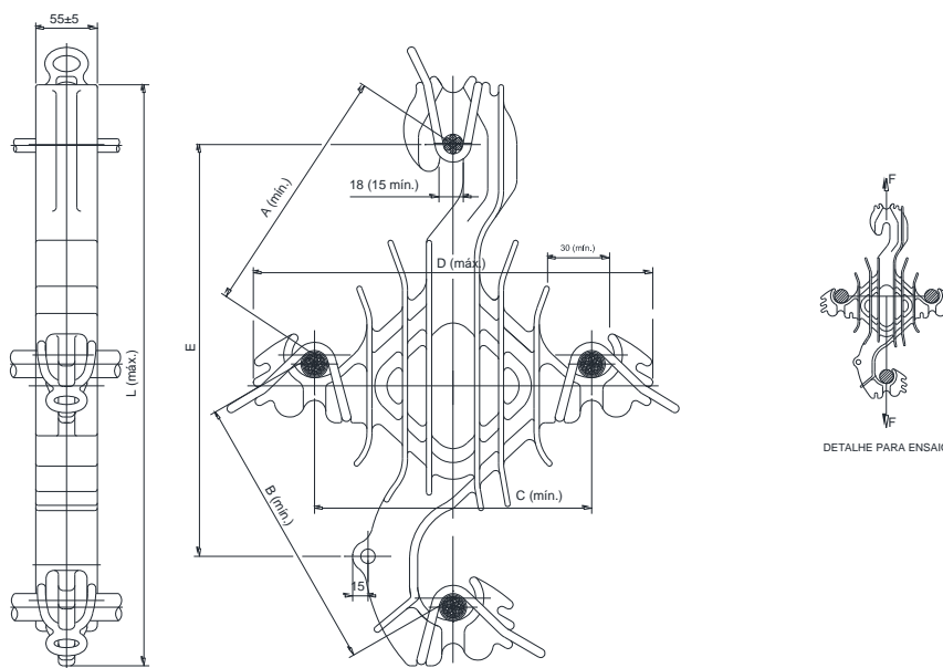
Figura 70 - Espaçador losangular
